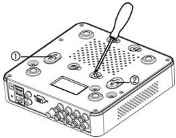
Рис. 1.1.2. Закрепление HDD
