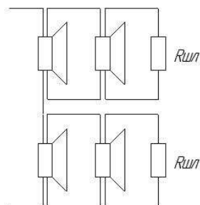
Подключение восьми акустических оповещателей Соната-5/1 40м, R_{\text{н}}=5\text{Вт} , R_{\text{вых}}=3,75\text{Вт} /оповещатель R_{\text{шл}} – резистор типа С1-4 0,25Вт 1,5кОм \pm 5\%
